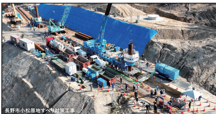
長野市小松原地すべり対策工事
